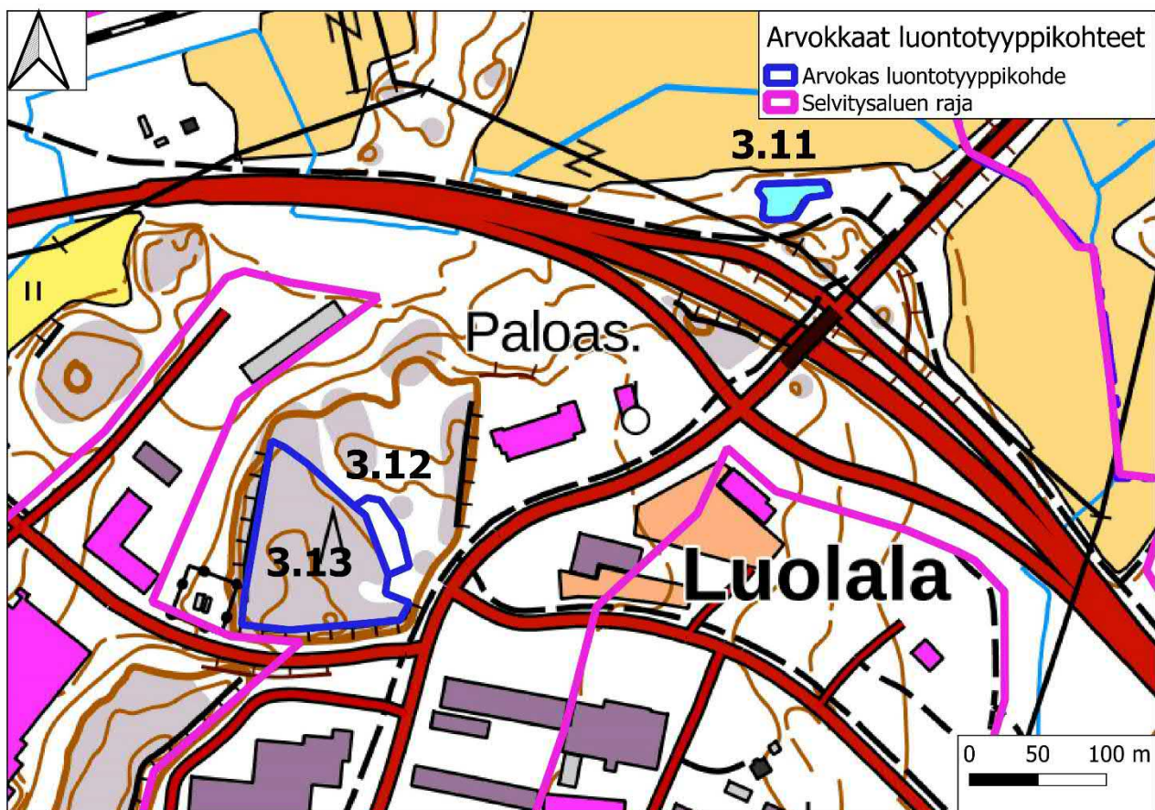
Kartta 5. Vanton eritasoliittymän lampi (3.11), Luolalankadun länsipuolen suolaikku (3.12), Luolalankadun länsipuolen kalliomännikkö (3.13).
