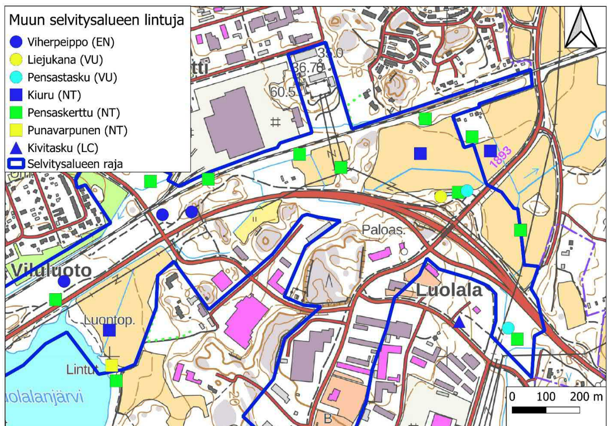
Kartat 7-8. Muun selvitysalueen pesimälintuja. (EN=erittäin uhanalainen, VU=vaarantunut, NT=silmälläpidettävä, LC=elinvoimainen)
