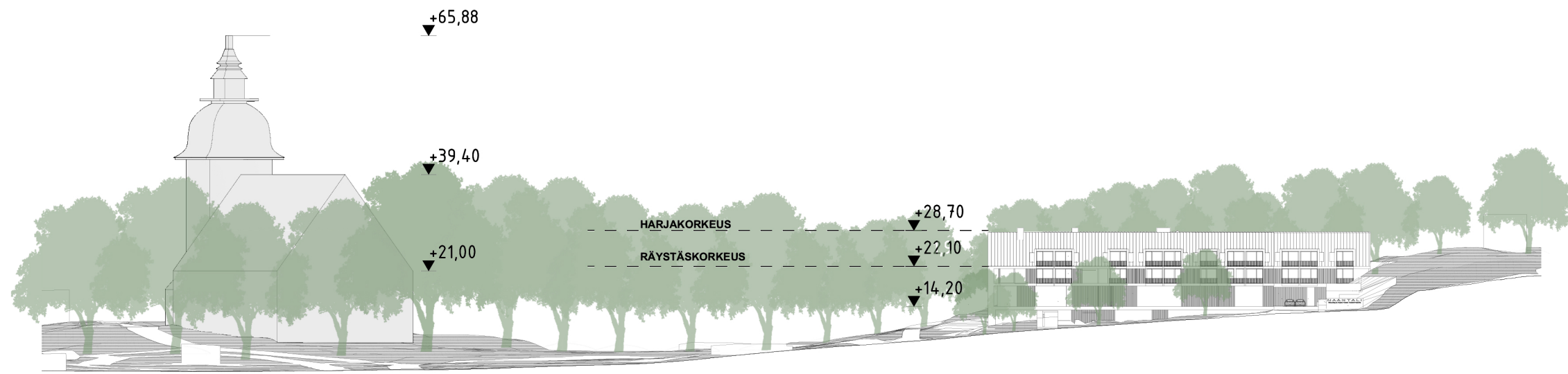
1:1000 ALUEJULKISIVU MAARIANKADULTA
